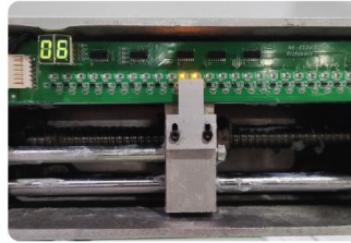
ระบบเปลี่ยนสีด้ายด้วยสวิตช์สูง ความเร็วสูง เปลี่ยนสีครบ 9 เข็มภายใน 1.2 วินาที ช่วยเพิ่มประสิทธิภาพงานปักหลายรูปแบบได้อย่างโดดเด่น
